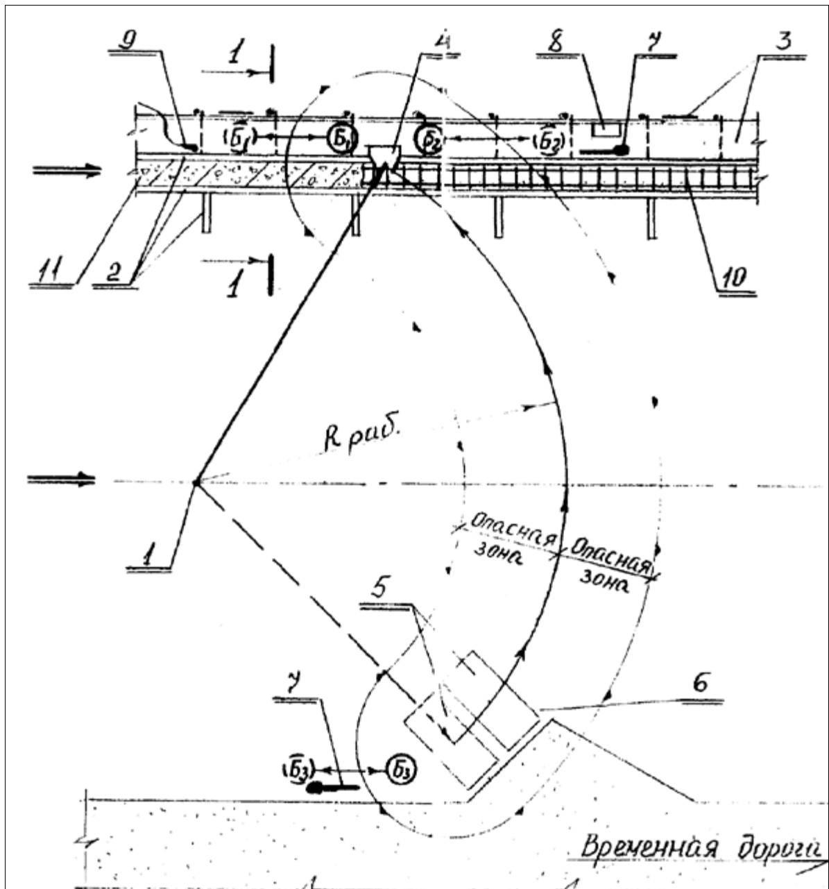
Рис.8. Схема подачи груза к рабочему месту
