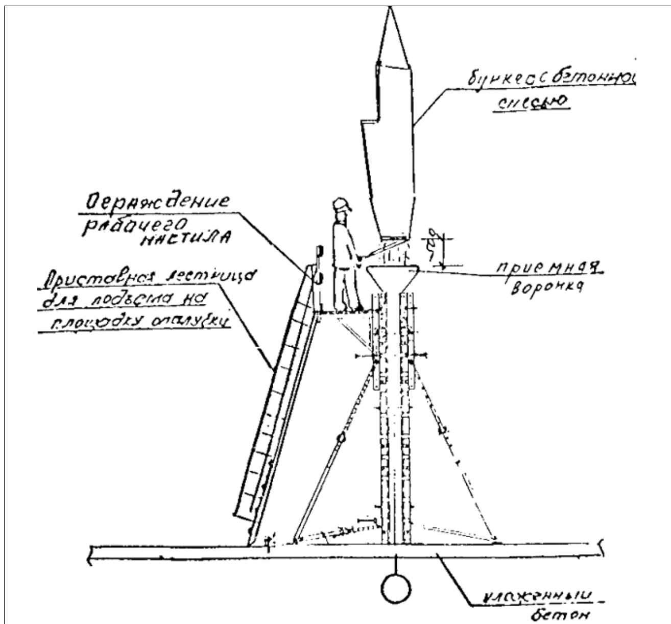
Рис.3. Укладка бетона в приемные воронки (лотки)
