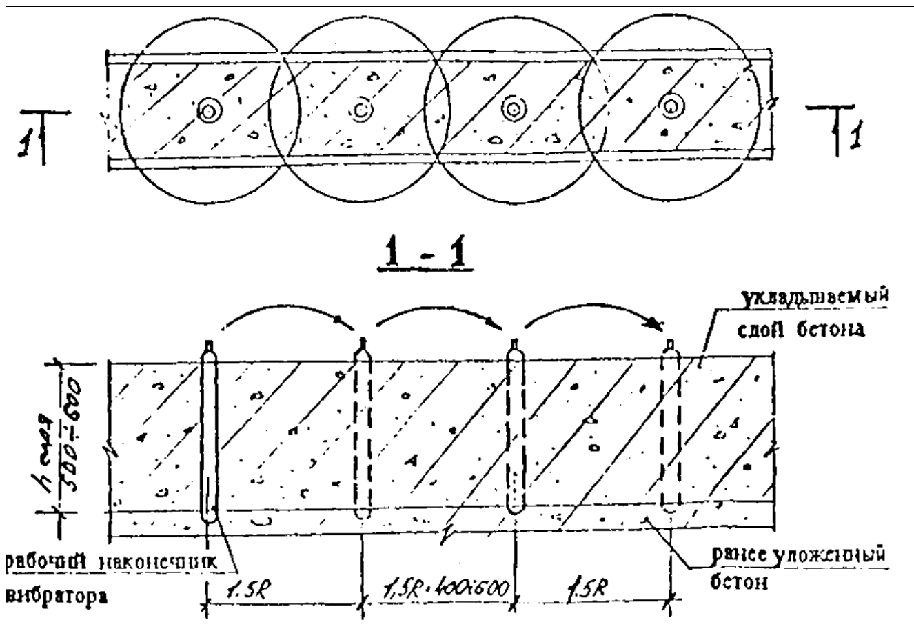
Рис.4. Схема уплотнения бетонной смеси глубинными вибраторами ИВ-47, ИВ-67
