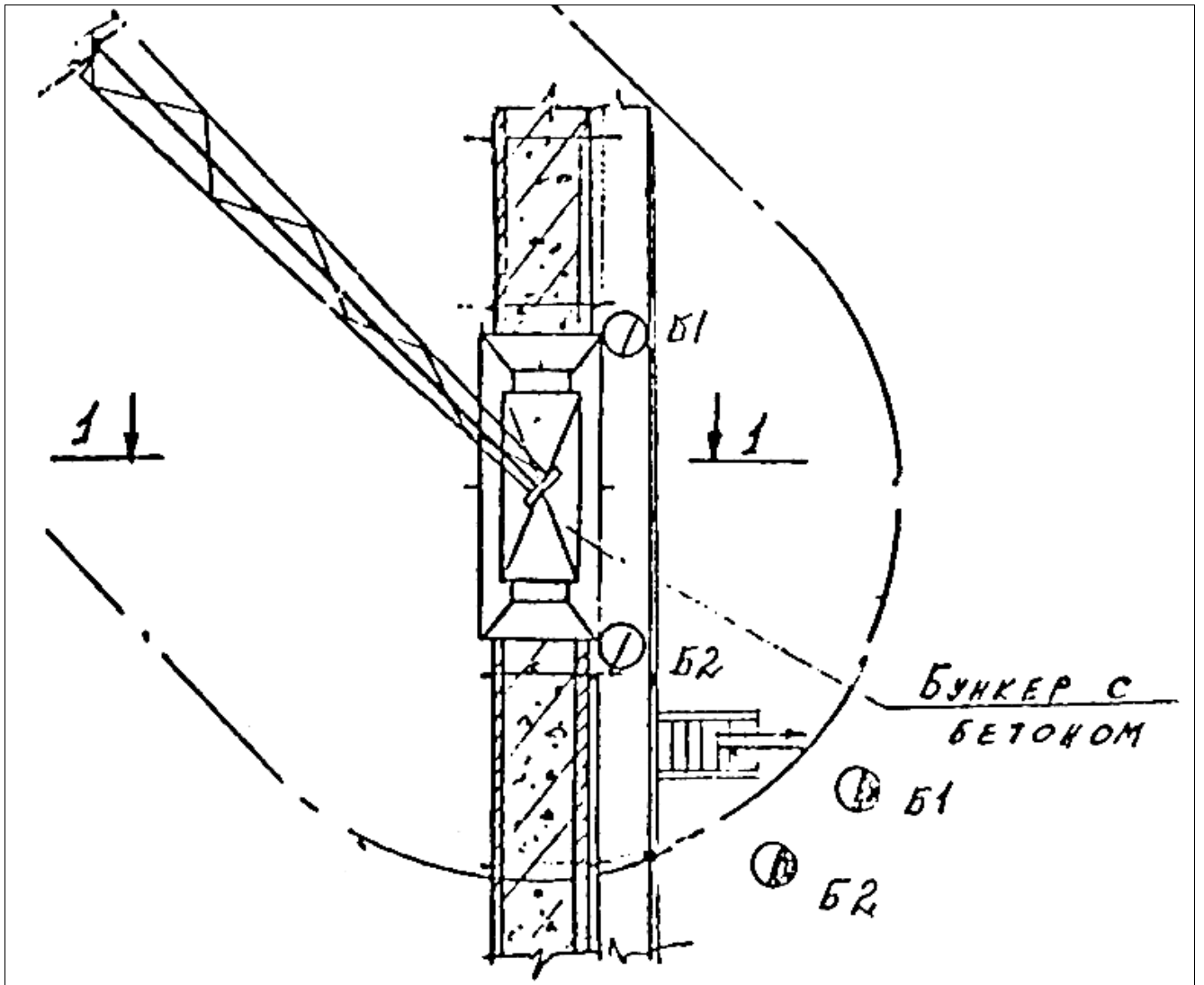
Рис.1. Подача бункера со смесью краном (фрагмент плана)
