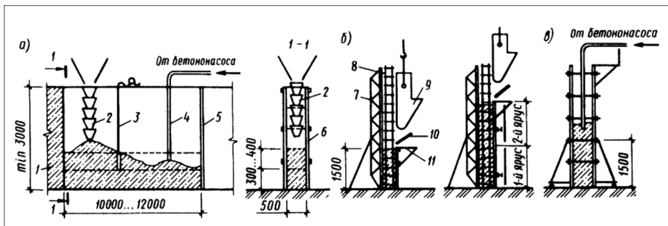
Рис.11. Укладка бетонной смеси в стены и перегородки:
