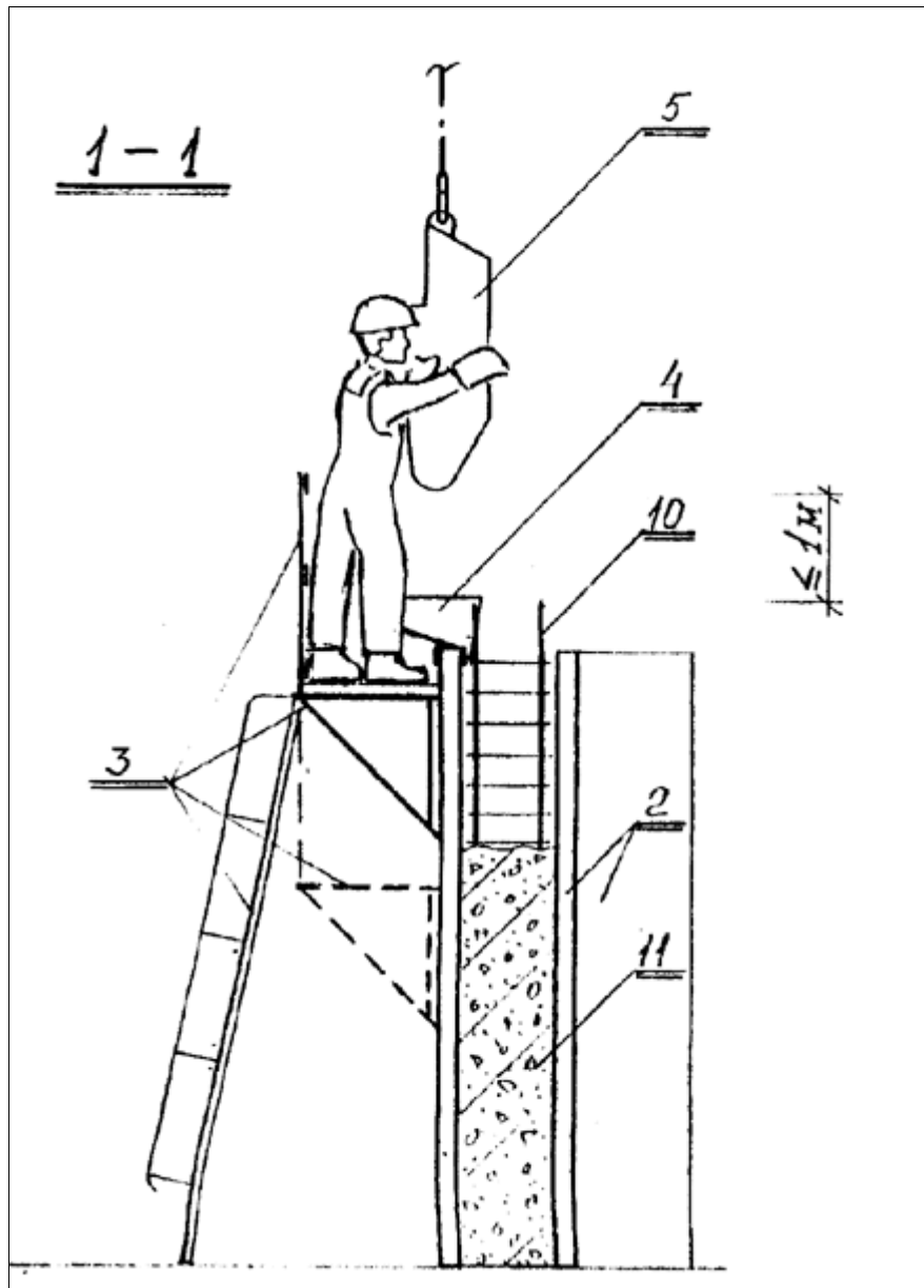
Рис.7. Прием раздаточного поворотного бункера с бетонной смесью
