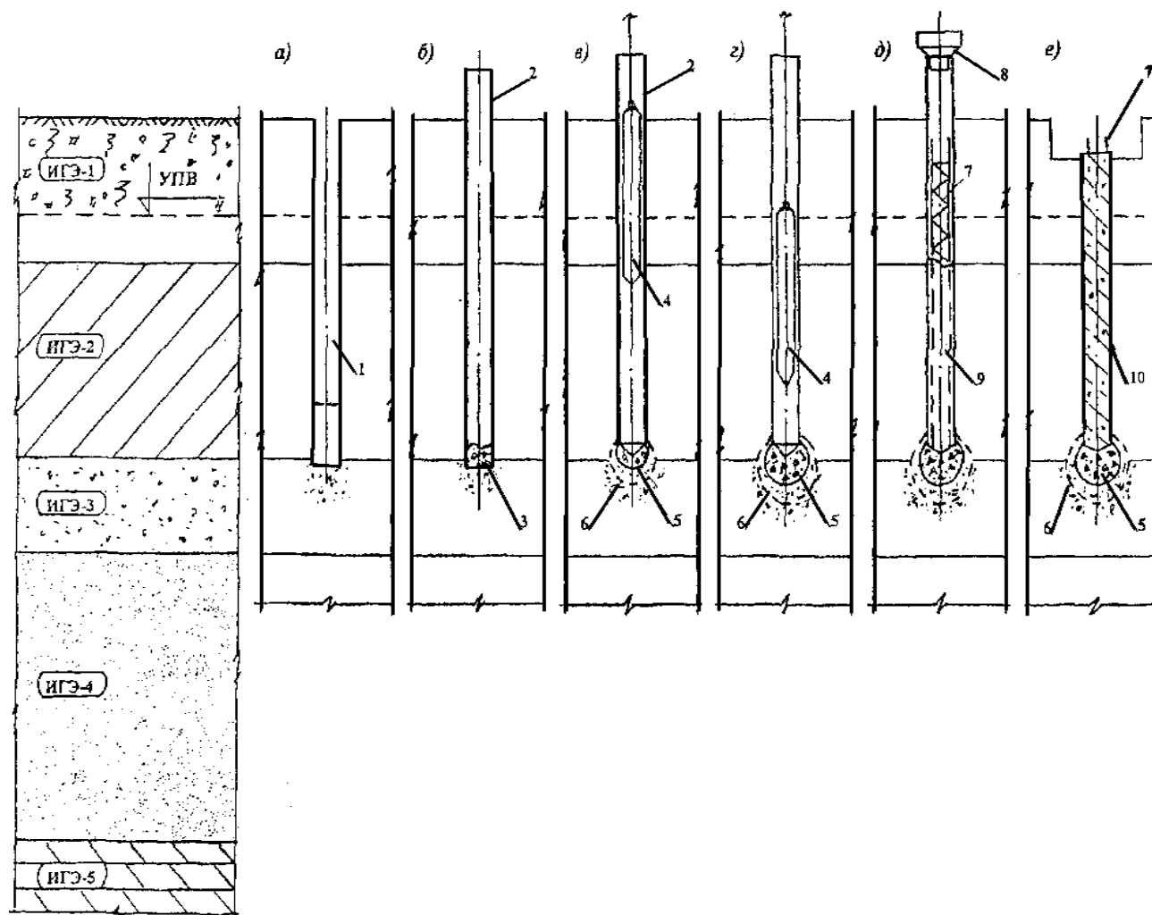
Рис. 1 Технологическая схема устройства буронабивной сваи (БСИу)
