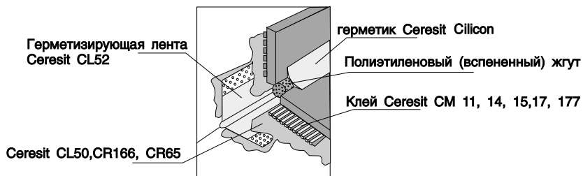
Рисунок 7 - Устройство деформационных швов.
