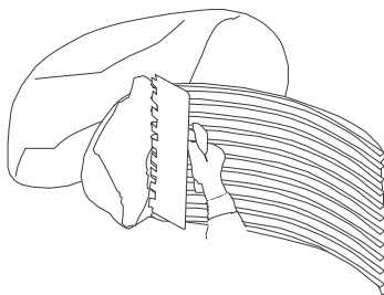
Рисунок 4 - Распределение растворной смеси зубчатым шпателем.
