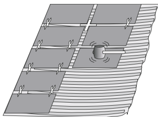
Рисунок 7 - Корректирование положения плитки с помощью резинового молотка.
