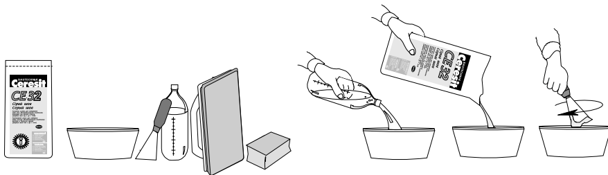
Рисунок 8 - Приготовление затирочной растворной смеси.
