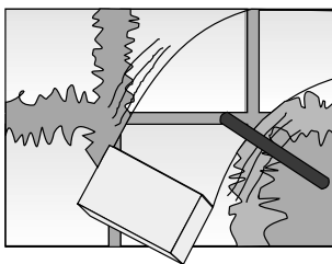
Рисунок 11 - Формование поверхности затирочной массы в швах.
