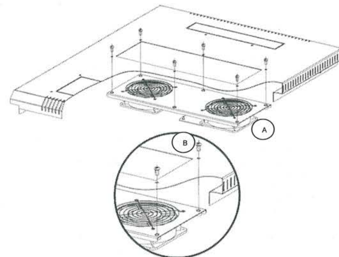
Рисунок 1. Установка потолочной вентиляторной панели
