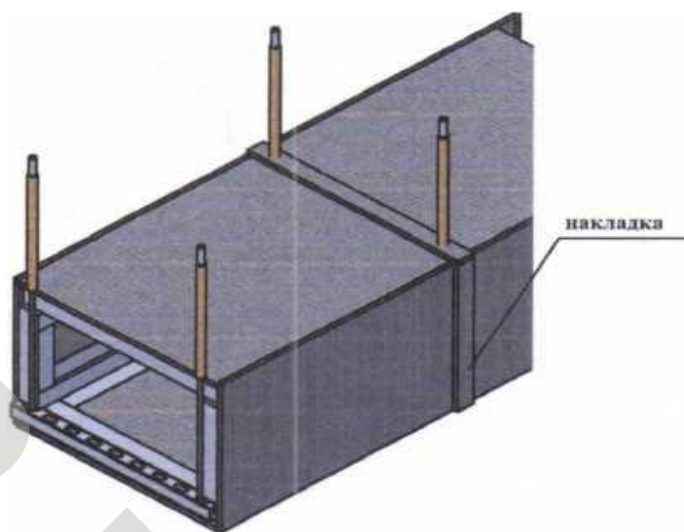
Рис. 3 Устройство накладок из плит на однослойную конструкцию ОКК.
